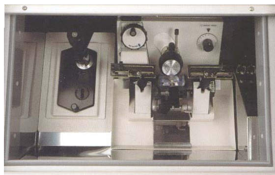
En la foto superior se muestra el micrótomos en el interior de la cámara. A su izquierda se ve el Congelador Rápido con los moldes para muestras y el disipador de calor.
