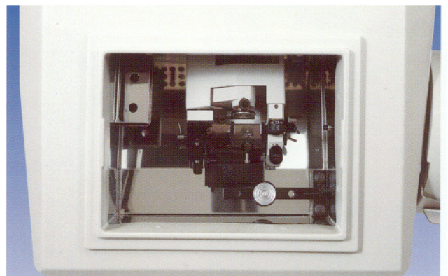
En la foto superior se muestra el microtomo en el interior de la cámara. A su izquierda se ve el Congelador Rápido con los moldes para muestras y el disipador de calor.
